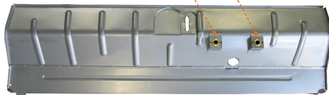
5200862 VOETENBAK -70 (zo origineel)
