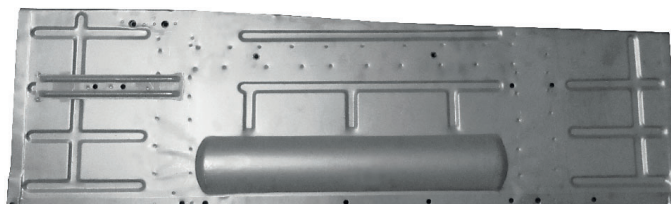
520903 VLOERPLAAT BINNEN RAND RALLYE LINKS
