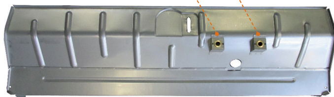
5200862 PLANCHER PEDALE -70 (comme originale) / BAGUES LAITON
