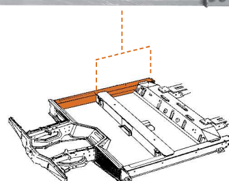
512982 SCHWINGTRÄGER RECHTS
