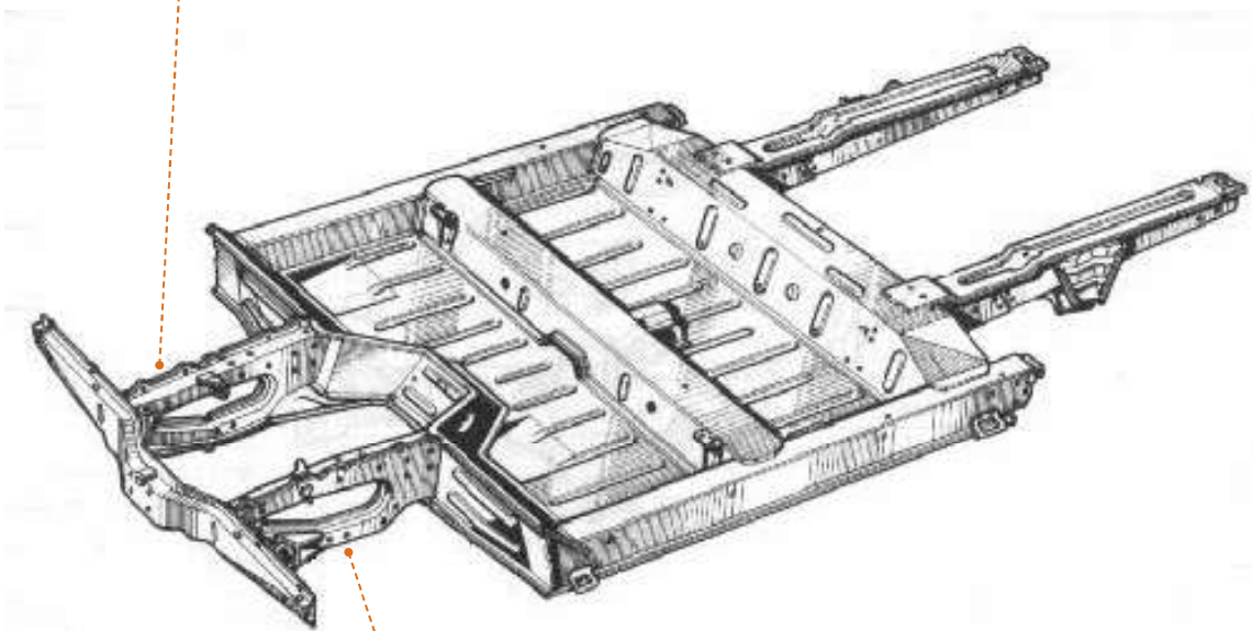
512895 MOTORTRÄGER RECHTS
