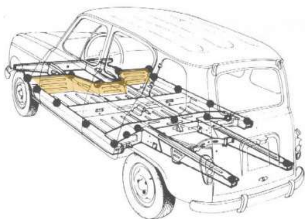
512584 PEDALBLECH
